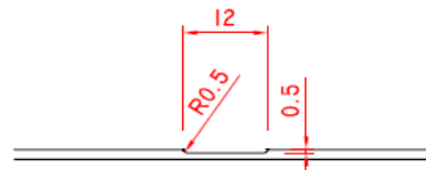
Type 20 (12 x 0,5 mm) Aluminium
